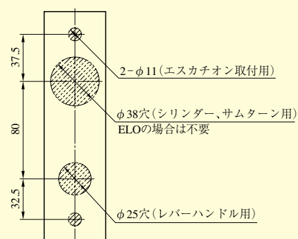
ELA15、16、17、30型を使用した場合の切欠 (ELOの場合はφ38穴が不要)
