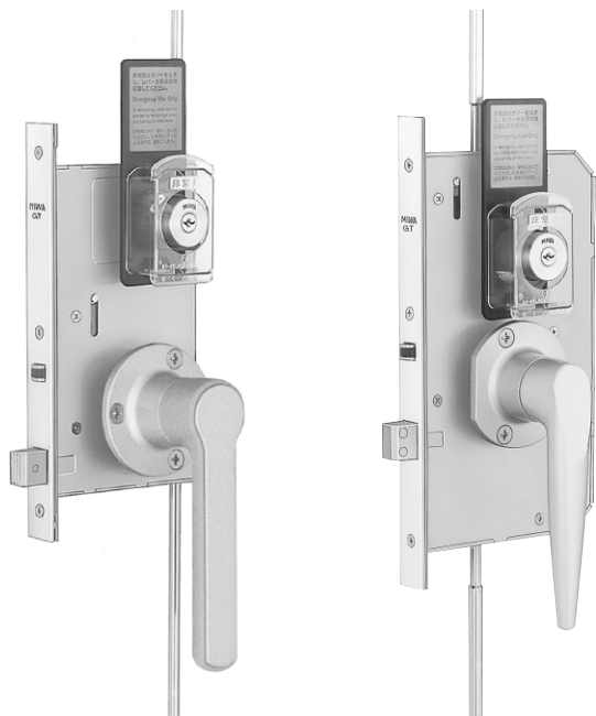
写真はU9GT6192-4E型 写真はU9GT5191-4E型
