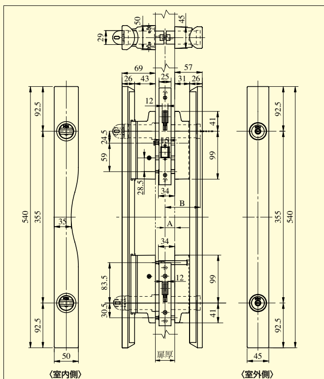
【外形図】
